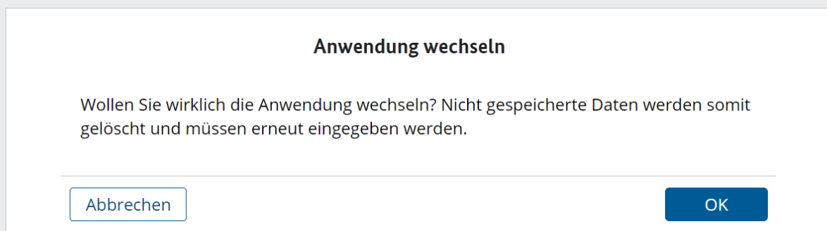
Abb. 2: Anwendung wechseln
